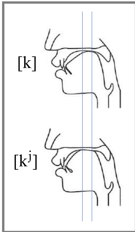
図1 口蓋化の例
